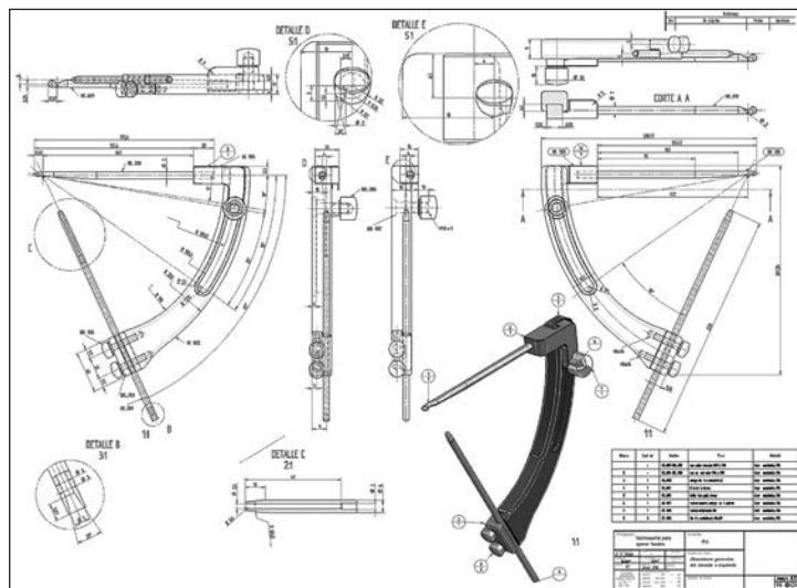
Figura 1. Diseño de la guía externa
